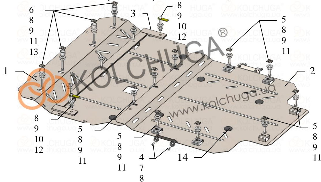
Схема сборки защиты радиатора, двигателя, КПП
